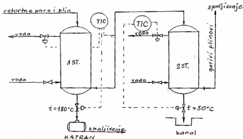
Slika 4. Odvajanje katraskih sastojaka kondenzacijom SDO-a u dva stupnja (Prijedlog I).
