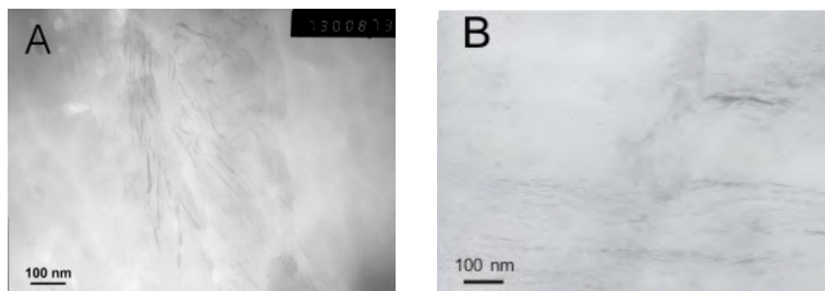
Slika 2. TEM snimke raslojenog PS nanokompozita s udjelom LDH-B od 2,5%. Na slici A prikazan je uzorak s polistirenskom matricom pri povećanju od 73.000 \times , a na slici B uzorak s kopolimerom PS-PMMA matricom pri povećanju od 56.000 \times .
